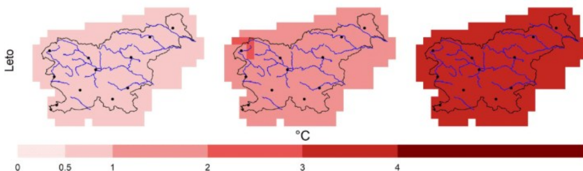
Slika 22: Sprememba povprečne temperature zraka po meteoroloških letnih časih in za celo leto v treh projekcijskih obdobjih glede na obdobje 1981–2010 za pesimistični scenarij izpustov (RCP8.5).
