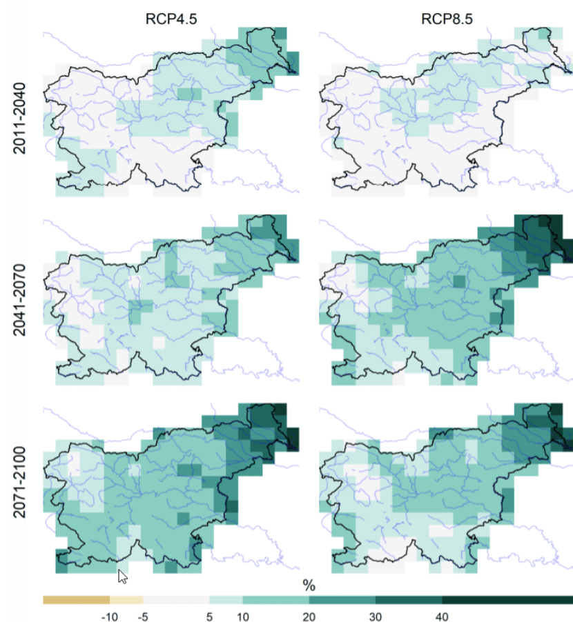
Slika 24: Spremembe povprečnega letnega napajanja podzemne vode za tri projekcijska obdobja in dva scenarija izpustov RCP4.5 (levo) in RCP8.5 (desno) glede na primerjalno obdobje 1981–2010
