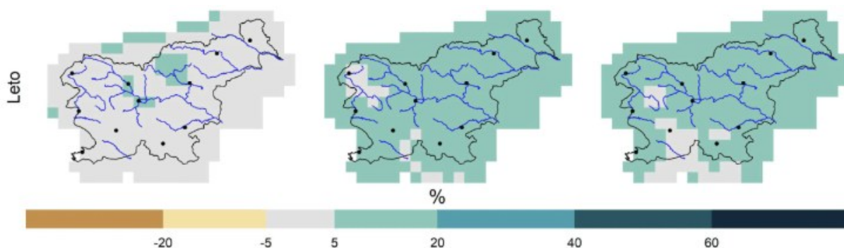
Slika 23: Sprememba povprečne višine padavin po meteoroloških letnih časih in za celo leto v treh projekcijskih obdobjih glede na obdobje 1981–2010 za pesimistični scenarij izpustov (RCP8.5)
