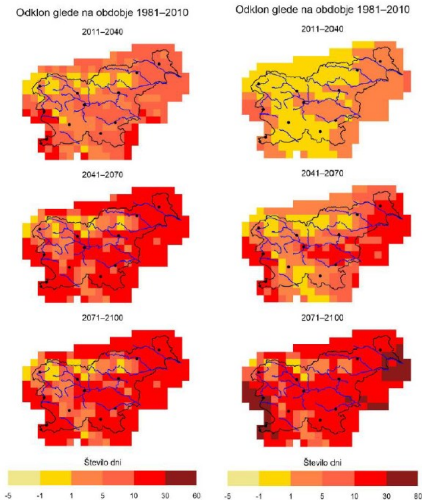
Slika 25: Število vročih dni in število tropskih noči glede na scenarij (RCP4.5)
